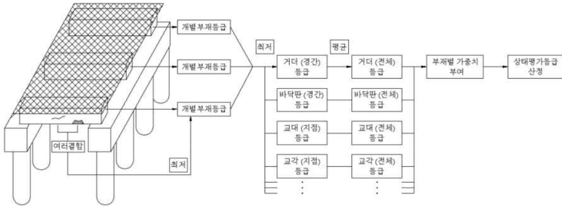
[그림 1.1] 전체 교량의 상태평가결과 산정 방법 예
